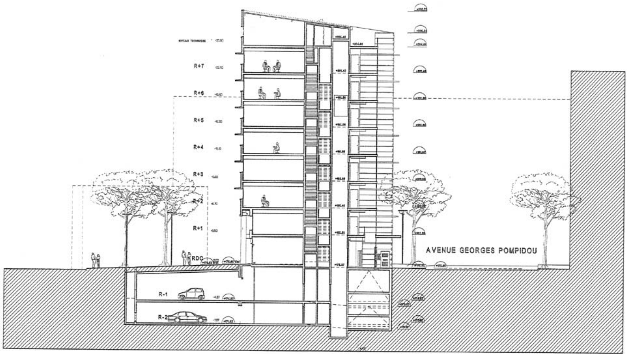
COUPE TRANSVERSALE
