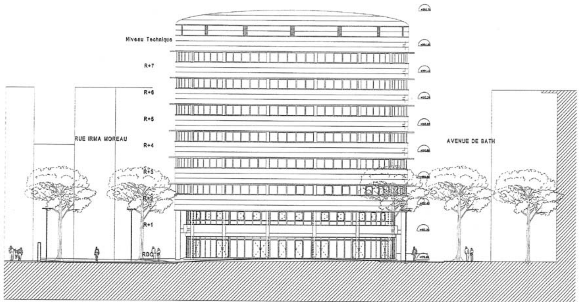
FACADE OUEST
