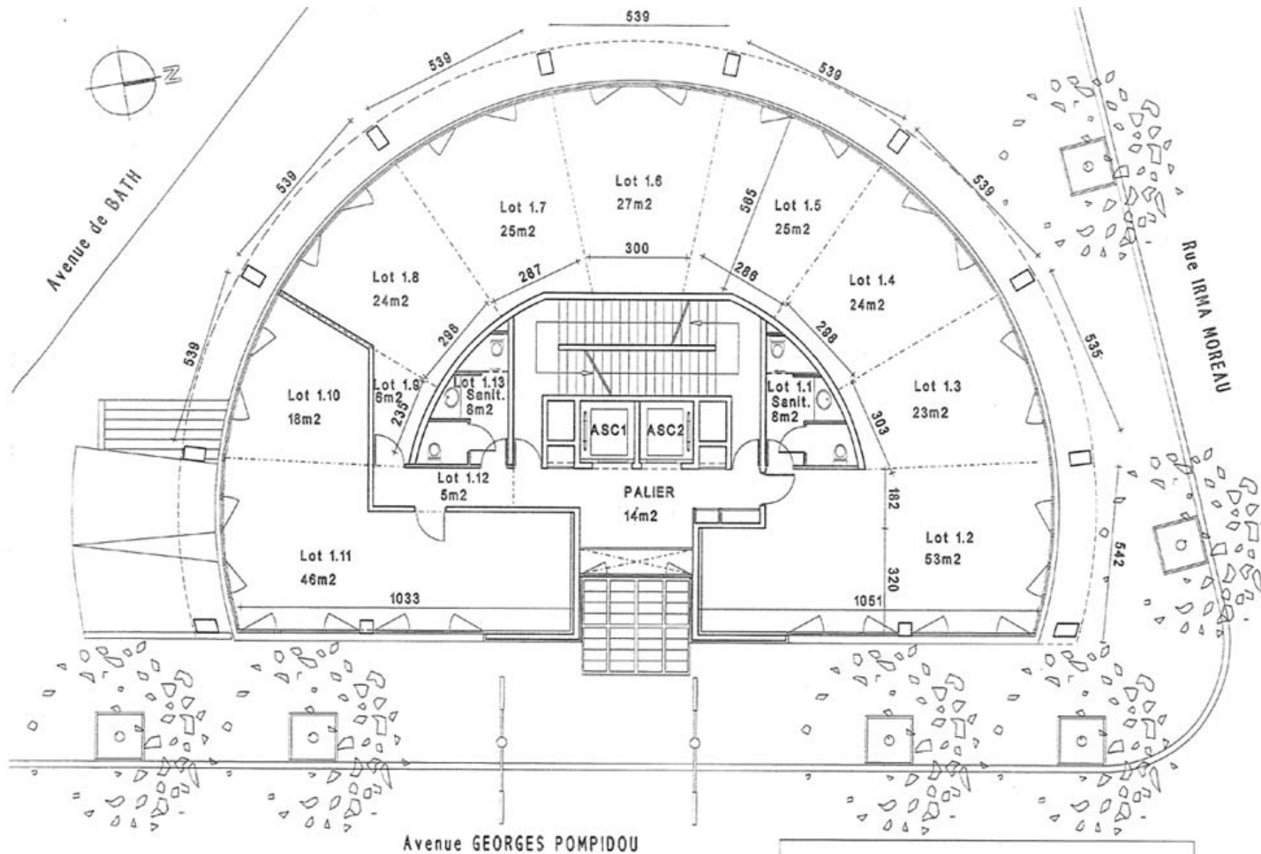
PLAN DU R+1 (+182.00)
