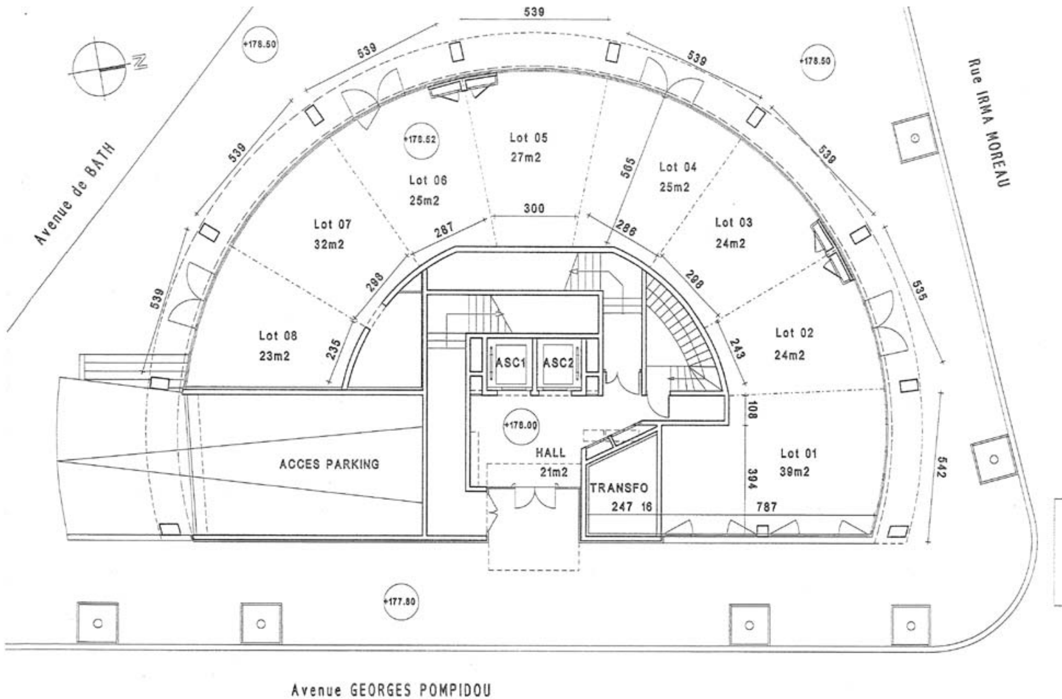
PLAN DU REZ DE CHAUSSEE
